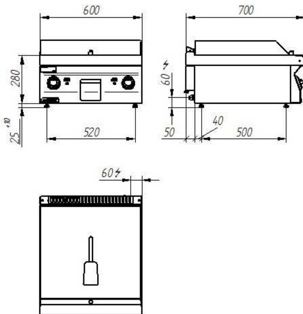
rys 3. Wymiary 700.PBE-600
